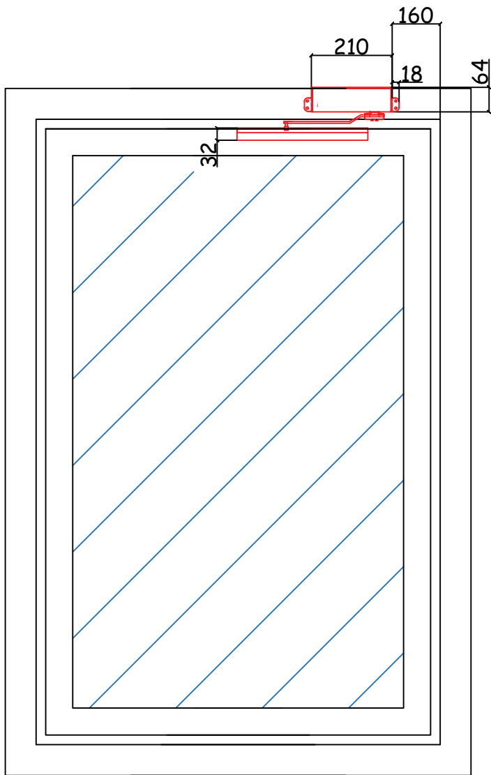
VISTA FRONTALE
